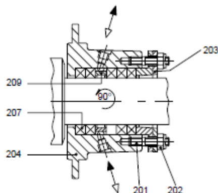
P3 сальник с набивкой с расположенным внутри кольцом уплотнительной камеры
